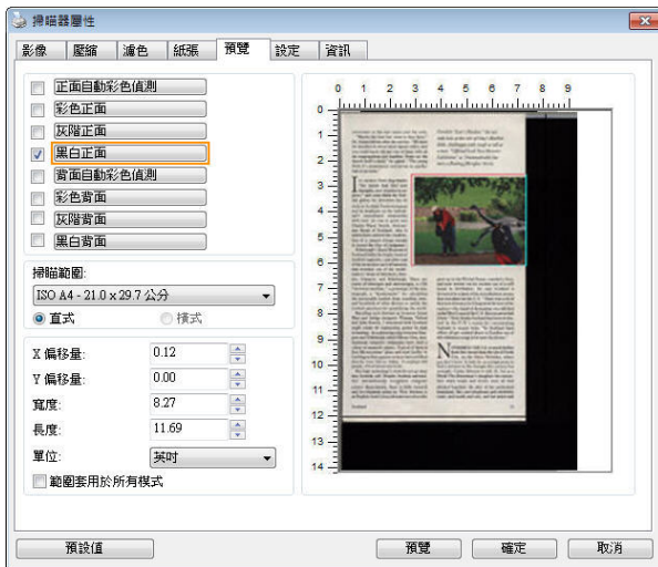
「預覽」頁簽
