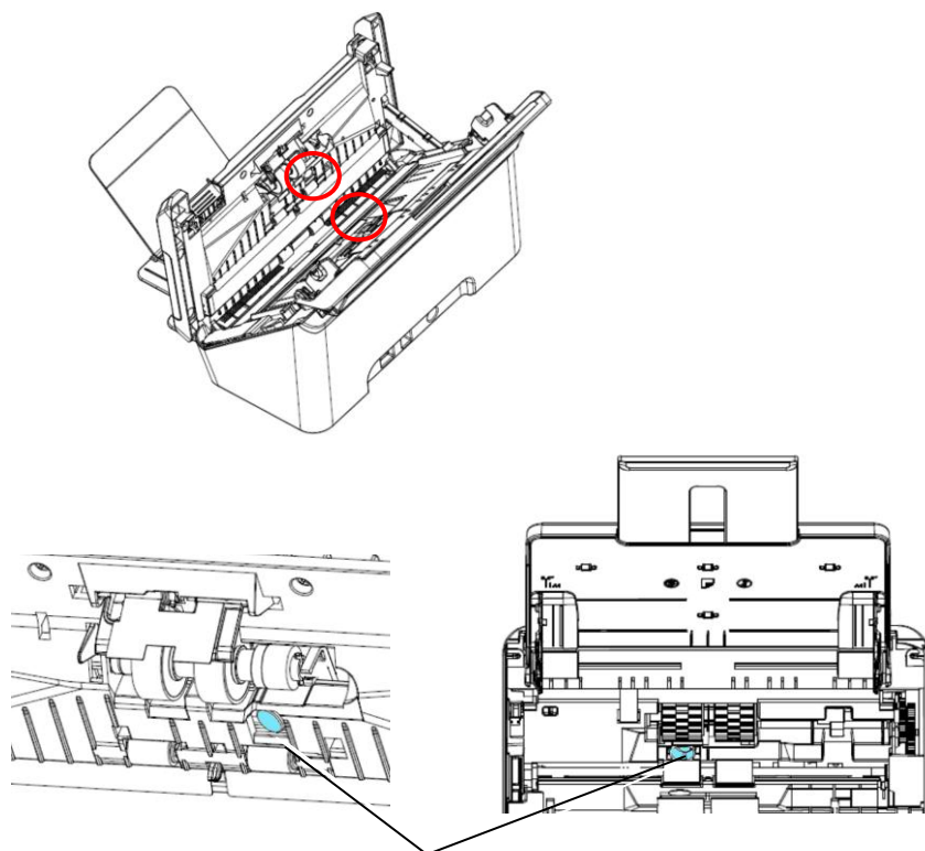
超音波センサー (Ultrasonic Sensors)
