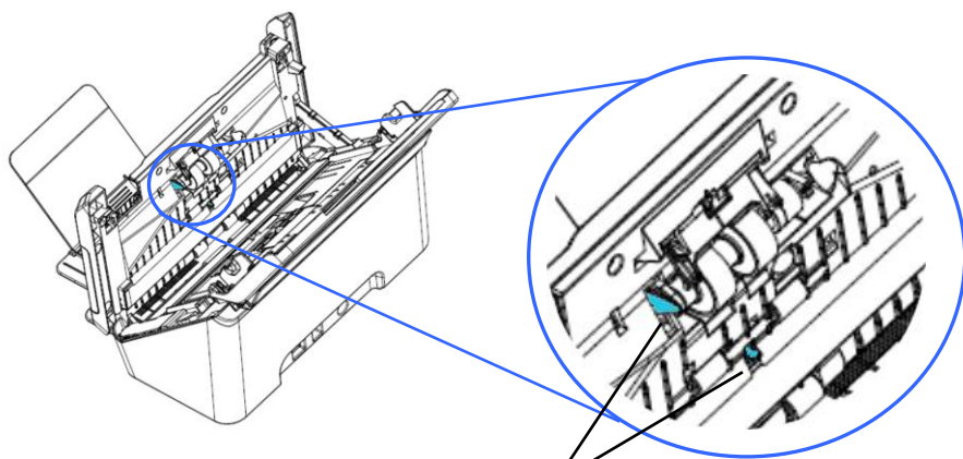
アームセンサー (Arm Sensor)
