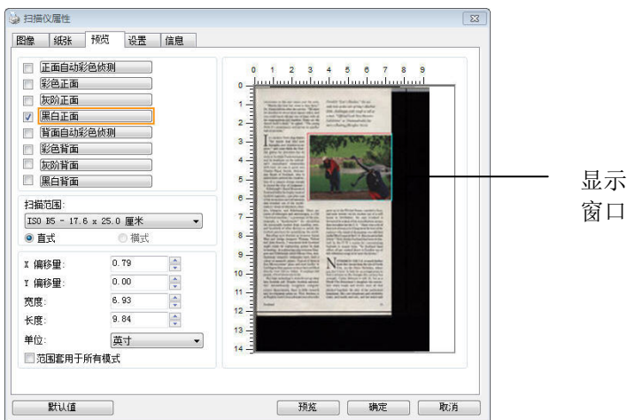
「预览」页签
