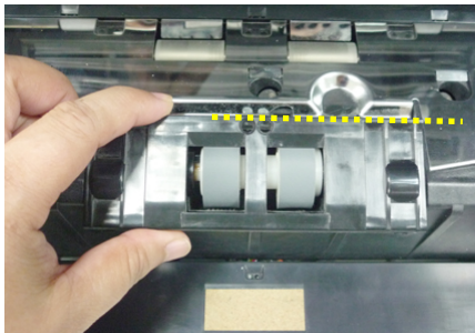
Coperchio del rullo di inversione
