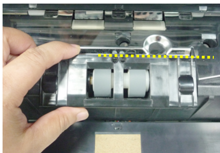
Pokrywa rolki odwracające
