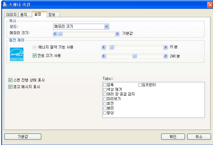
설정 탭 대화상자
