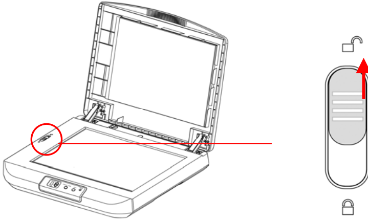
圖2-1 開啓掃描器鎖定開關
