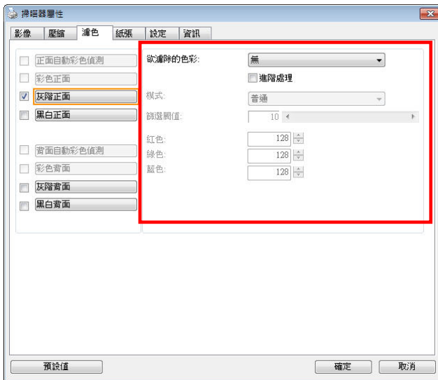
「濾色」對話框
