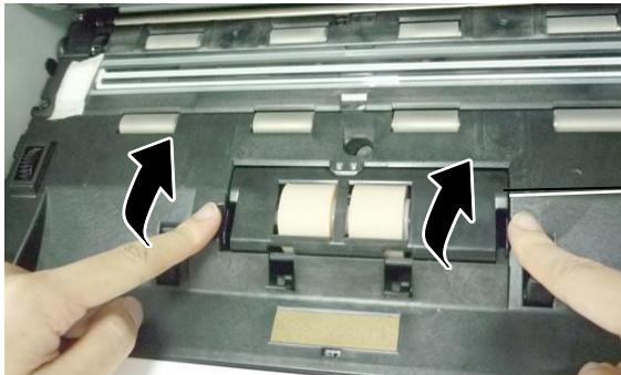
Abdeckung der Umlenkwalze
