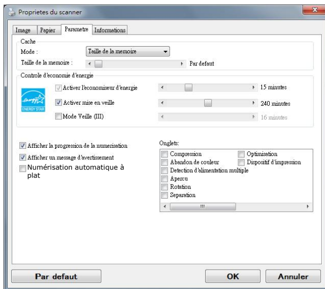
La boîte de dialogue de l'onglet Paramètre
