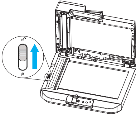
그림 2-1 스캐너 풀기
