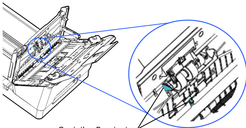
Czujnika Ramienia
