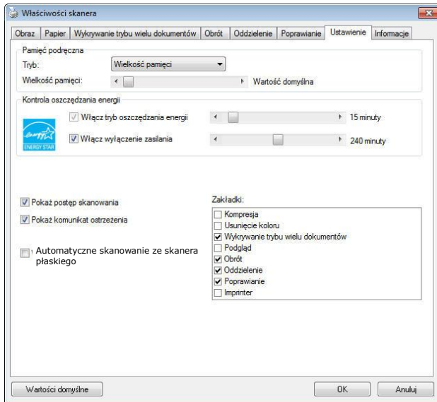
Okno dialogowe zakładki Setting (Ustawienia)
