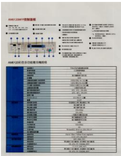
Brightness (Jasność): -50
